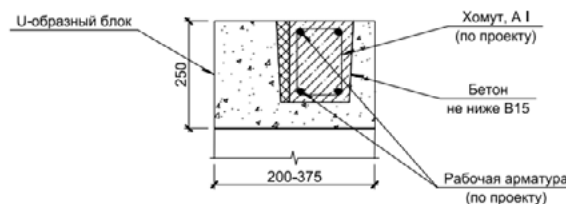
е) Простая U-образная перемычка
